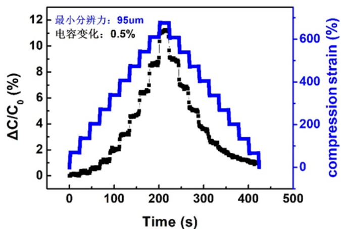
图 1-1 传感器分辨力
