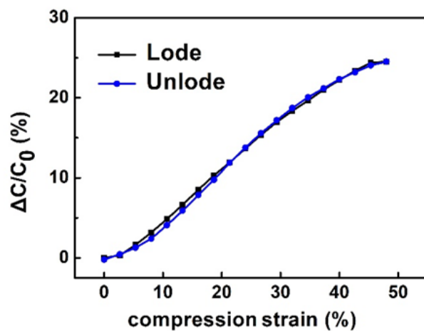
图 1-3 位移应变曲线
