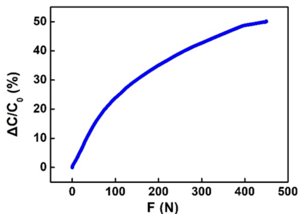
图 1-2 压力应变曲线
